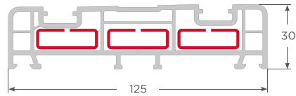
Marco corredera
