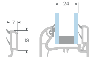
Tapa canal
