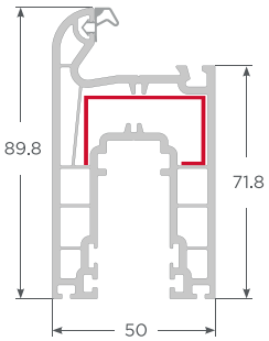
Hoja corredera
